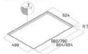
Foro d'incasso per montaggio flushtop Cut out flush mounting
