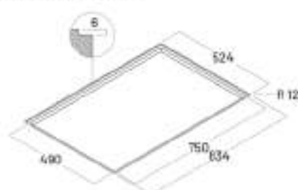
Foro d'incasso per montaggio filato Cut out flush mounting
